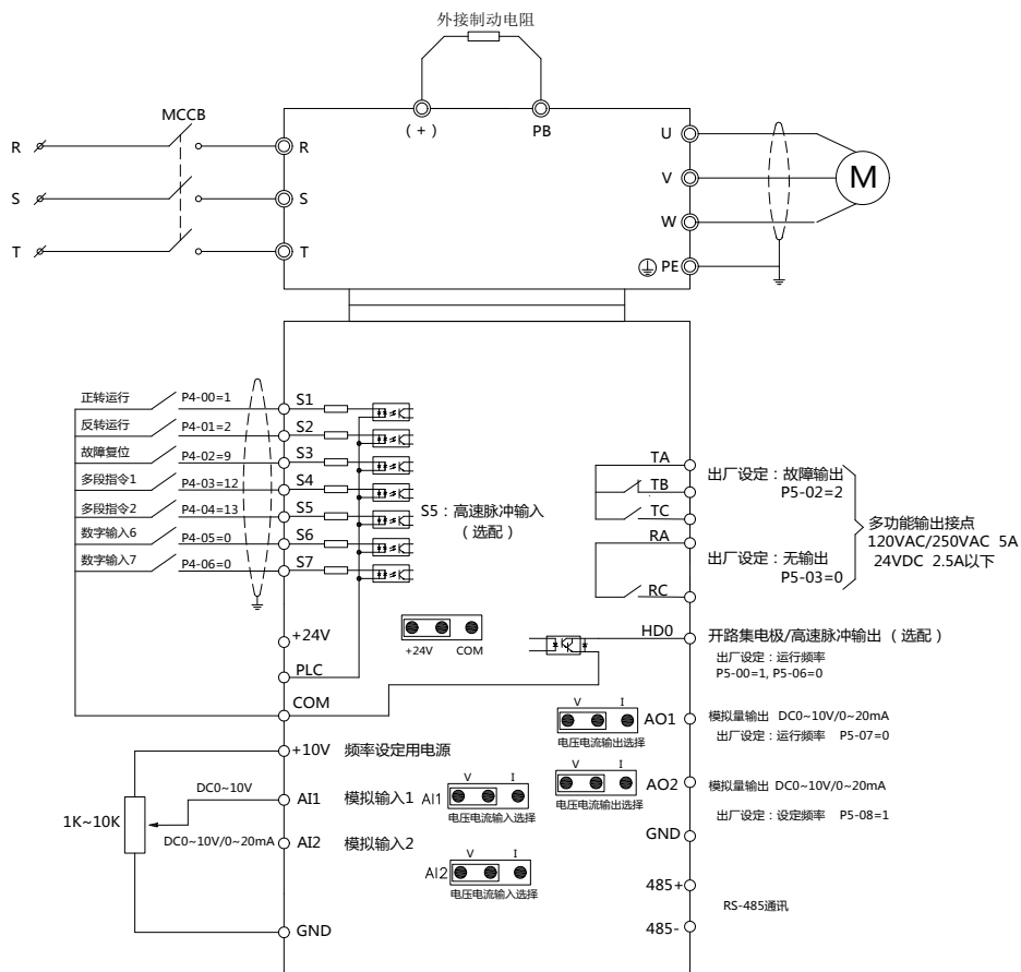
图 3-4 标准接线图
